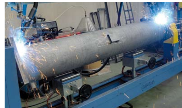
Automatic welding machine / Saldatura automatizzata
